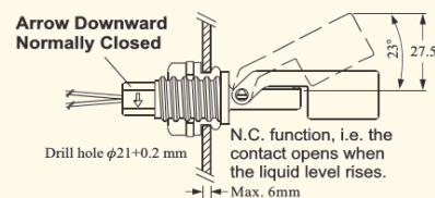
Mini Float Level Switch FineTek FCH21 $ 28.00
